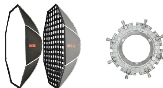
KE-150专业八角柔光箱/柔光箱格栅 Octagonal softbox/Grid #1.07.051119 #1.07.051204 φ150cm
